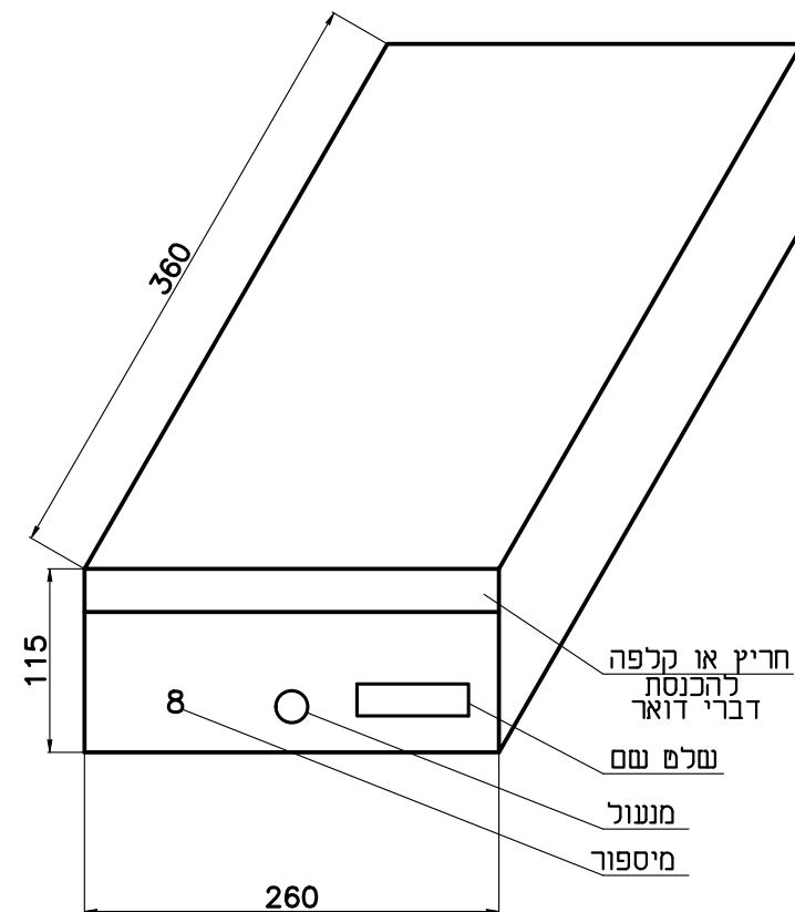
מידות תא
