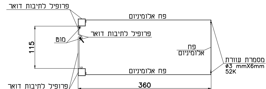
חתך אנכי
